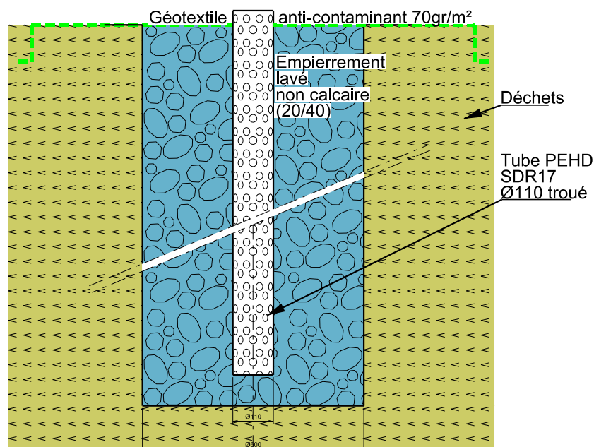
Coupe schématique d'un puits
