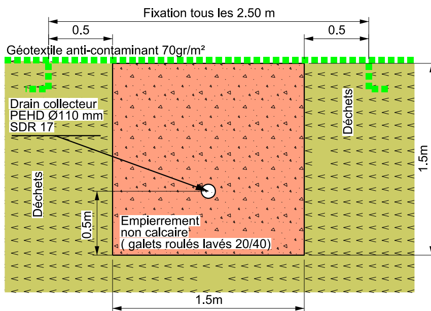
Coupe schématique d'une tranchée
