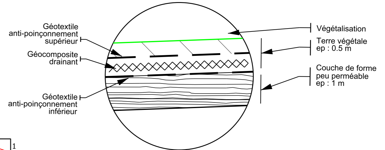
Figure 2.24 : Coupes - Détails
